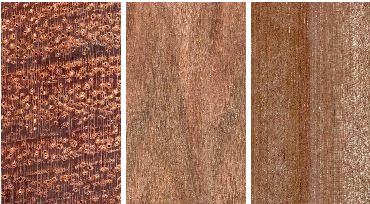
Angelim vermelho ( Dinizia excelsa ): Querschnitt ca. 10x, tangentielle und radiale Oberfläche (natürl. Größe)
