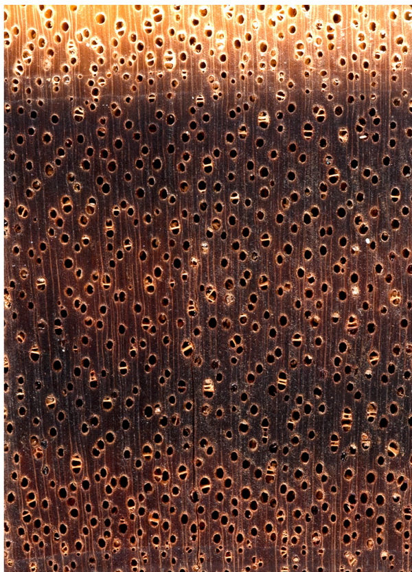
Mangium ( Acacia mangium ): Querschnitt (ca. 12-fach) und radiale Oberfläche (natürliche Größe)
