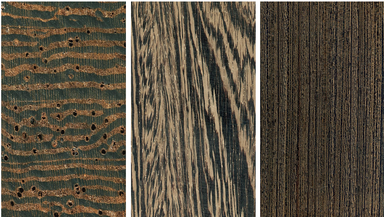
Wengé ( Millettia laurentii ): Querschnitt (ca. 12x), tangentielle und radiale Oberfläche (natürliche Größe)
